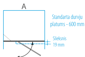
KREISAJĀ PUSĒ MONTĒJAMAS DURVIS
